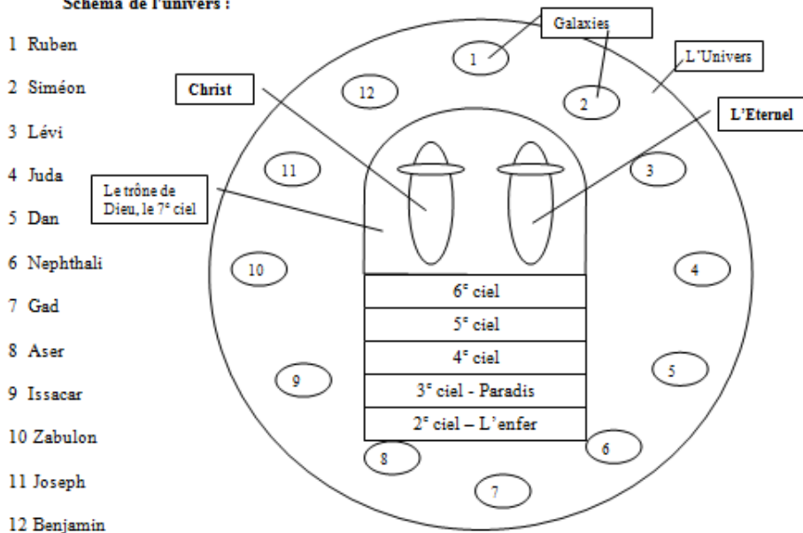
Schéma de l'univers :
